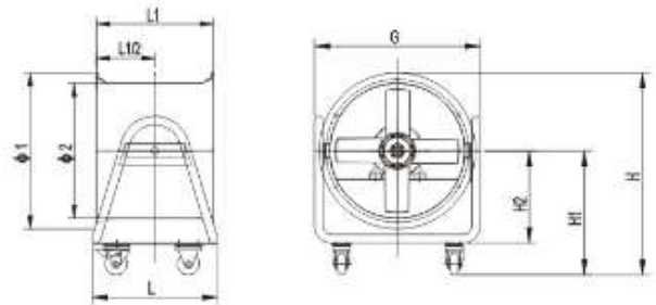
安装尺寸图 Mounting dimensions
